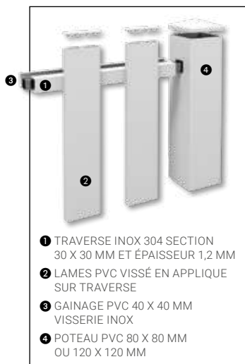
Coloris 1015 FT - Dimensions maxi entre poteaux : 1800 mm
