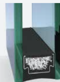
INTERCALAIRE THERMIX
