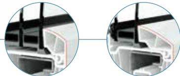
PARCLOSE TRIPLE ET DOUBLE VITRAGE
